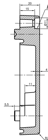
SECTION A-A
