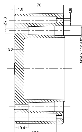
SECTION D-D
