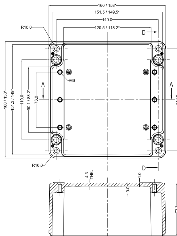
SECTION A-A
