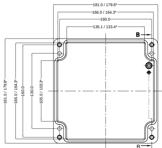
LID
